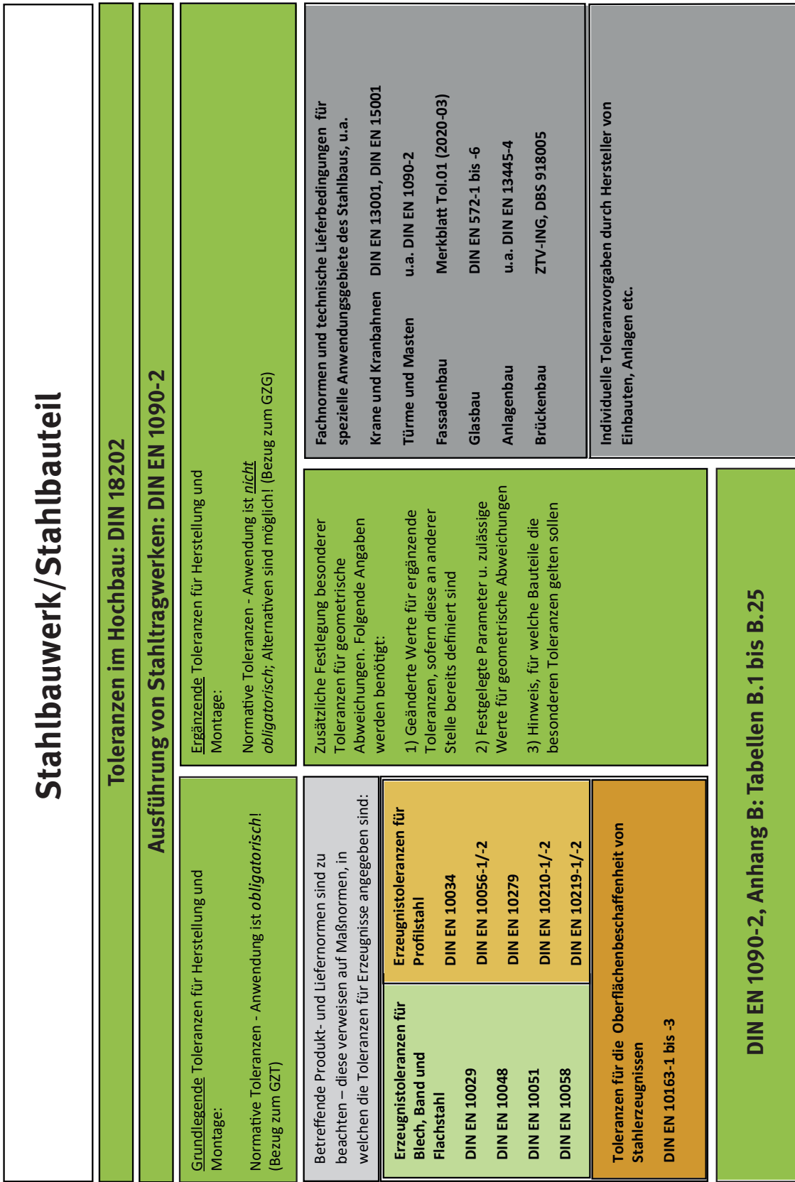
Schaubild: Systematik der Toleranznormen im Stahlbau
