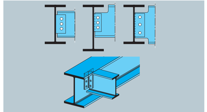
Bild 3: Trägeranschlüsse mit und ohne Ausklinkung
