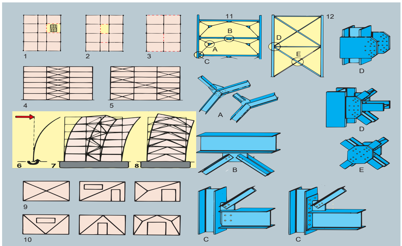
Bilder 1 bis 12: Anordnung und Tragverhalten von Verbänden; Ausführung von Verbandsstäben und -anschlüssen
