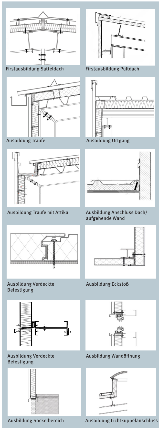
Bild 4: Sandwichelemente: Anschluss- und Stoßdetails
