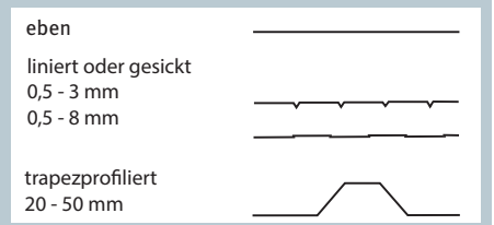
Bild 3: Geometrie der Deckblechprofile
