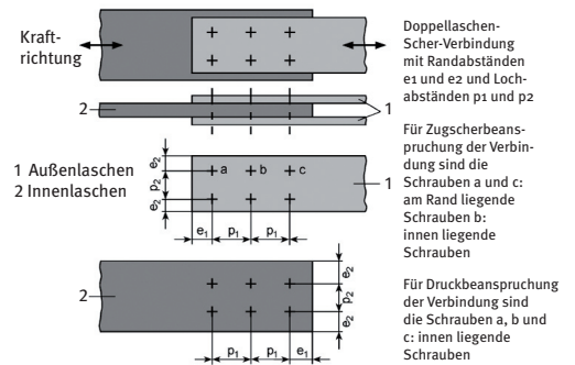
Bild 3 Doppellaschen-Scher-Verbindung mit Rand- und Lochabständen
