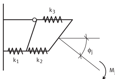
Bild 12: Federmodell eines unversteiften geschweißten Träger-Stützen-Anschlusses [2]
