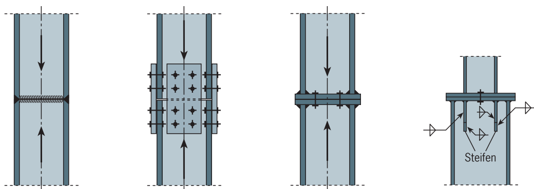
Bild 3: Stützenstöße [5]
